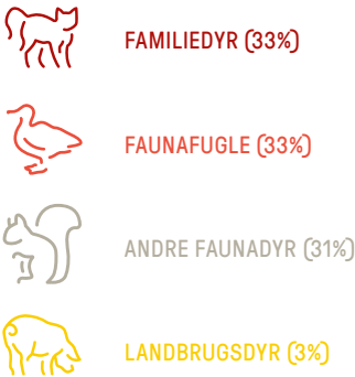
FIGUR 2 Fordelingen af sager i 2020 fordelt på dyregrupper
